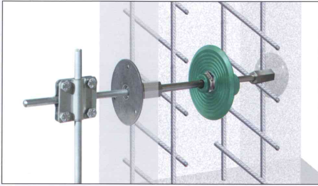
RONDO für Blitzschutz
