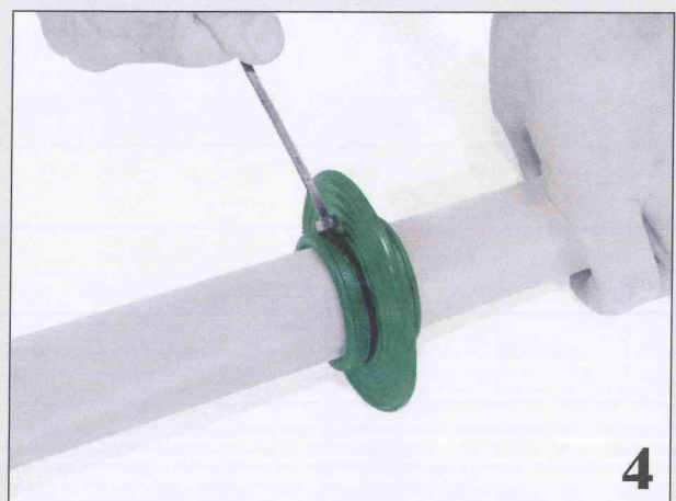
Festes Anziehen der beiden Spannbänder von Hand
