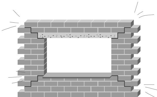
Murfor® unter der Fensterbank beugt Risschäden an dieser Stelle vor.
