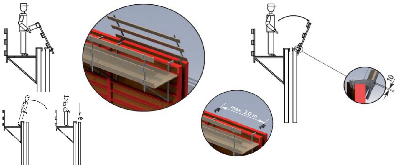
Während der Montage sind Geländerhalter und Bretter zur Betonierbühne geneigt
