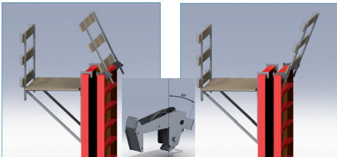
Während der Montage sind Geländerhalter und Bretter zur Betonierbühne geneigt
